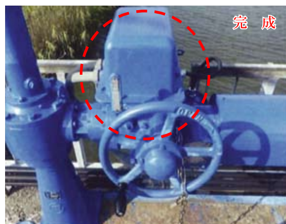
2号樋門
